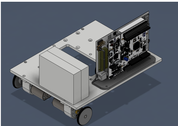
Abbildung 13: PES-Board und Akku
